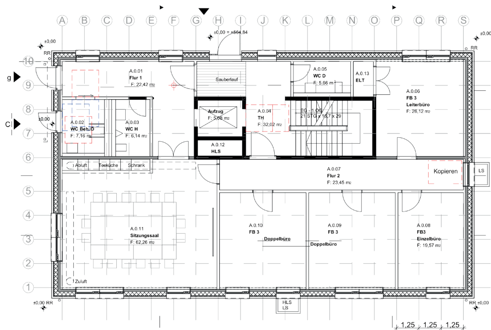
Grundriss Erdgeschoss
