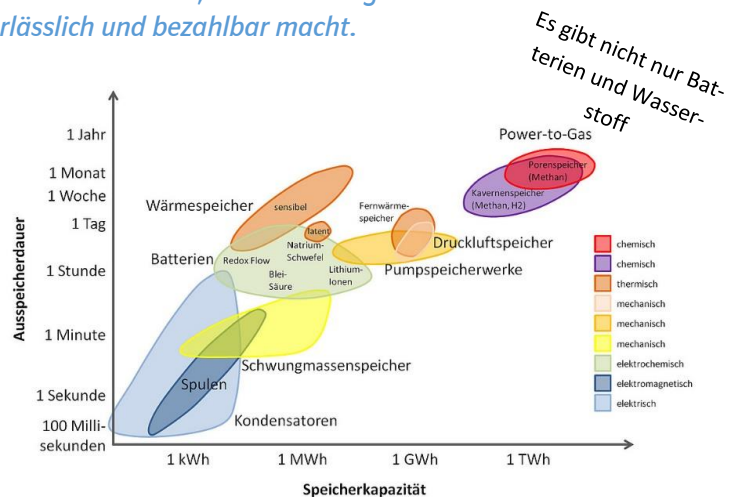
Abb. 1: Speicherkapazität und Ausspeicherdauer verschiedener Speichertechnologien im Überblick. Quelle/Copyright: Greenhouse Media GmbH, reproduziert nach Sterner, Stadler, Energiespeicher-Bedarf, Technologien, Integration, Springer-Vieweg 2014), https://www.energie-experten.org/erneuerbare-energien/oekostrom/energiespeicher Copyright: www.energie-experten.org Hamburg
